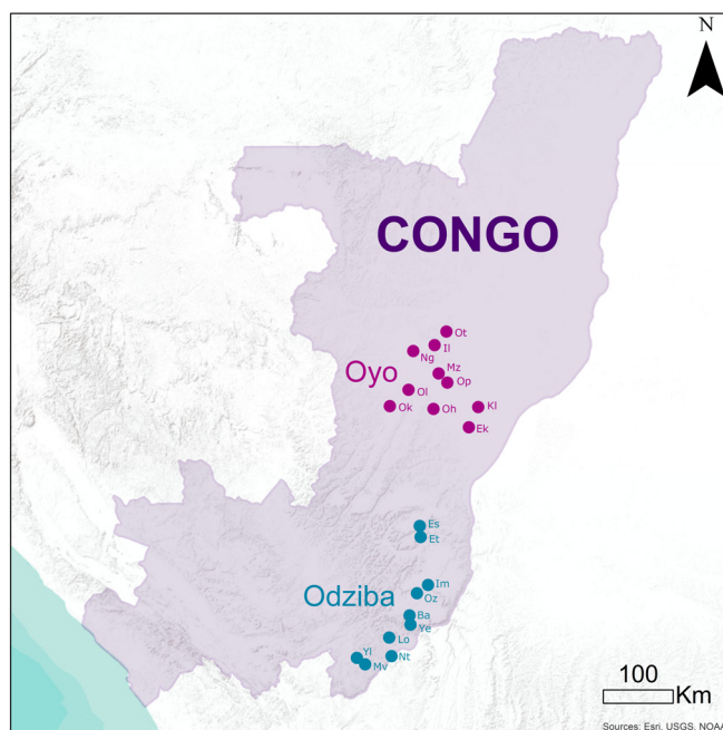
Fig. 1. Localisation des sites d'étude et abréviations des noms des villages. Site d'Odziba (Bambou mingali: BA; Essoua: ES; Etsouali: ET; Imbama: IM; Loumou: LO; Mvoulou mamba Sud: MV; Ntoula: NT; Odziba: OZ; Yie: YE; Yala mvounga: YL). Site d'Oyo (Ekongo: EK; Illebou Ondongo: IL, Koli: KL, Moundzeli: MZ; Ngoko: NG; Ohouri: OH; Okouesse: OK; Olongonen: OL; Opokania: OP; Otende: OT).
